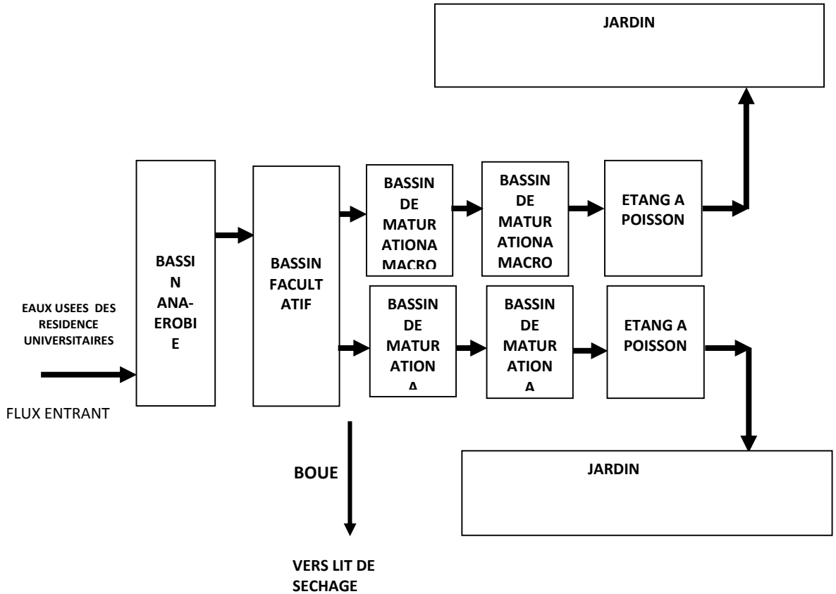
Figure 2 : Plan schématique de la station pilote
